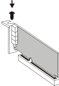
Рис. 7. Установка платы Ольха-14 в разъем материнской платы ПК
