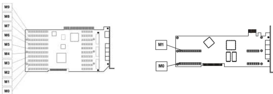
Рис. 6 Места для мезонинов на платах ОЛЬХА-14P Ольха-14LPX, Ольха-14LPE
