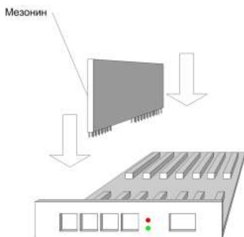
Рис.4 Вертикальная установка мезонинов
