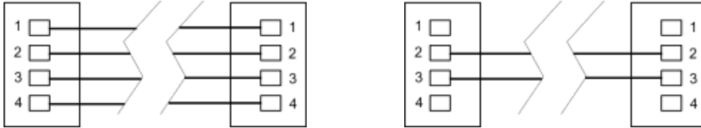
Рис. 11 Стандартный телефонный кабель
