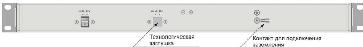
Рис. 32. Вид задней панели изделий MM-502RC-UNI-DCH
