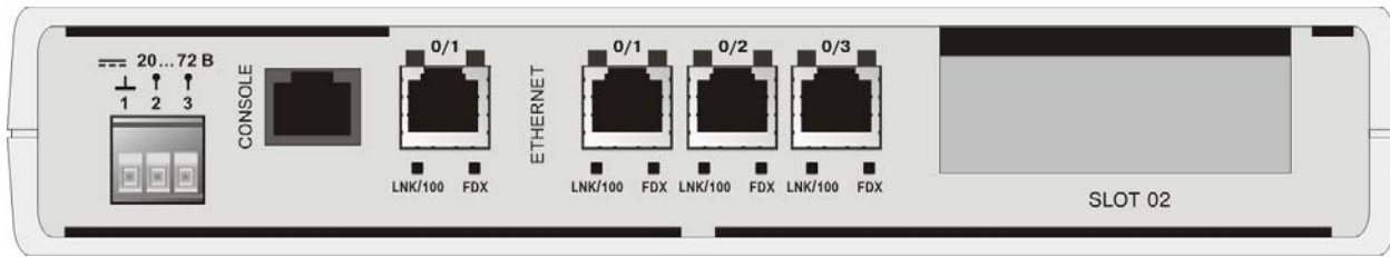
Рис. 27. Вид задней панели изделий MM-205x настольного исполнения с питанием от сети постоянного тока
