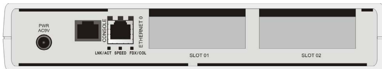
Рис. 21. Вид задней панели изделий MM-201x, MM-202x, MM-211x и MM-212x настольного исполнения с питанием от сети переменного тока
