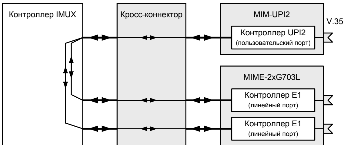
Рис. 15. Передача данных V.35 через два потока E1
