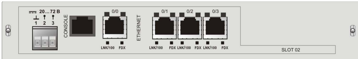
Рис. 29. Вид задней панели изделий MM-205x для установки в конструктивы P-12 и P-510 с питанием от сети постоянного тока
