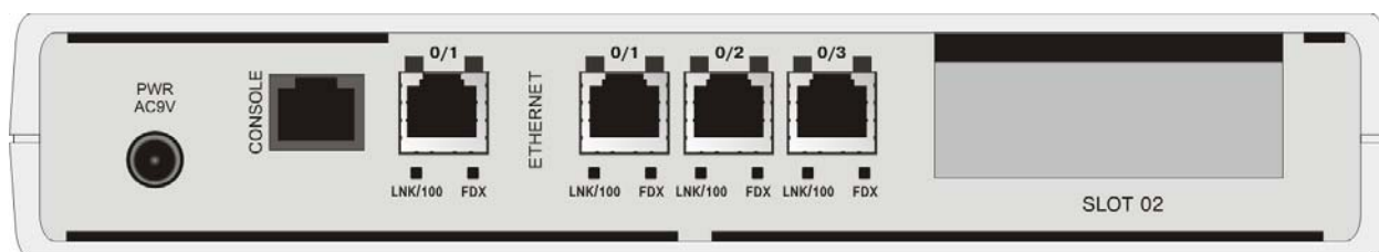
Рис. 26 Вид задней панели изделий MM-205x настольного исполнения с питанием от сети переменного тока
