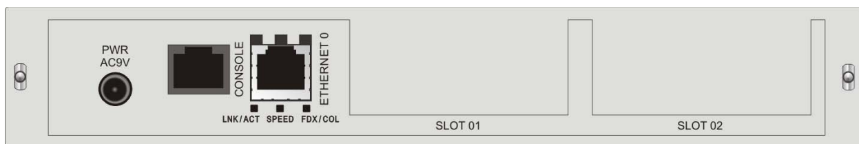
Рис. 23. Вид задней панели изделий MM-201x, MM-202x, MM-211x и MM-212x для установки в конструктивы P-12 и P-510 с питанием от сети переменного тока
