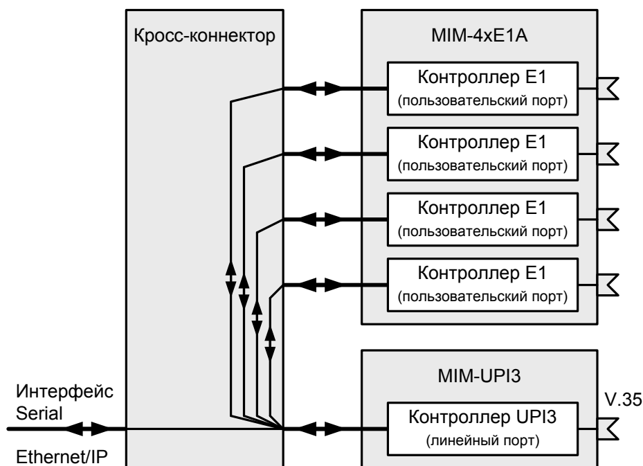
Рис. 13. Передача данных Ethernet/IP и четырёх потоков E1 через канал V.35
