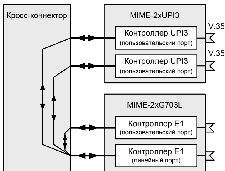
Рис. 8. Мультиплексирование данных V.35 и E1 в канал E1
