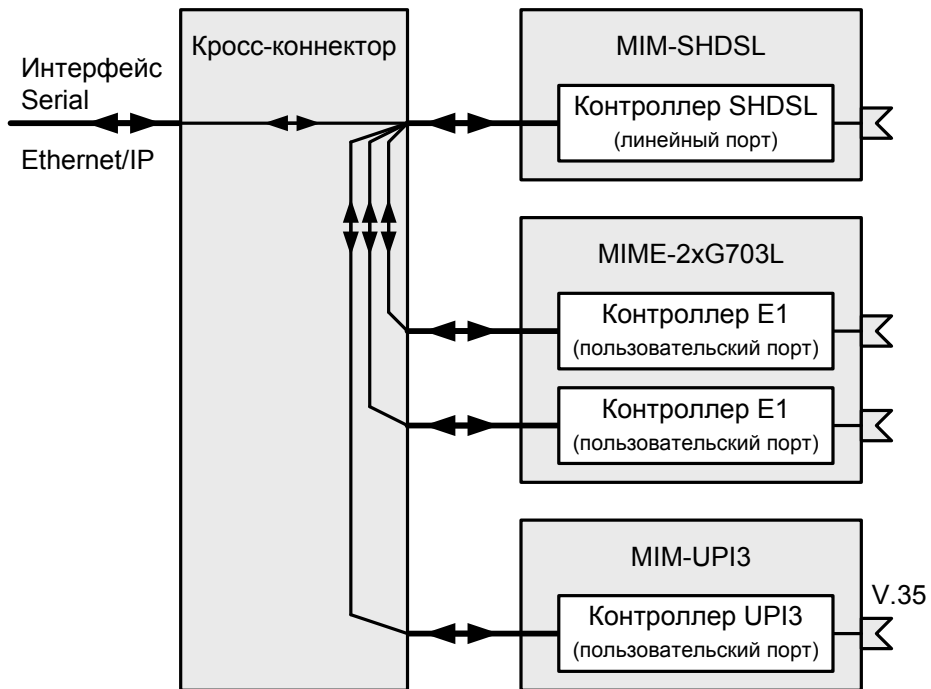
Рис. 12. Передача данных Ethernet/IP, V.35 и E1 через канал SHDSL
