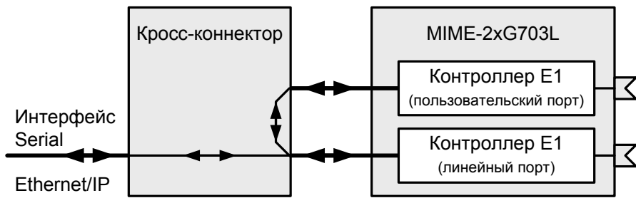
Рис. 10. Передача данных Ethernet/IP через выбранные таймслоты потока E1 в режиме извлечения — вставки
