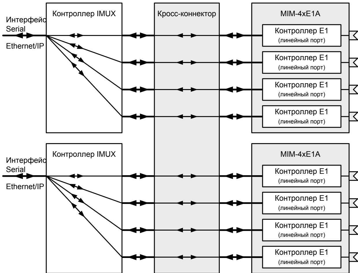
Рис. 14. Передача данных Ethernet/IP через четыре потока E1
