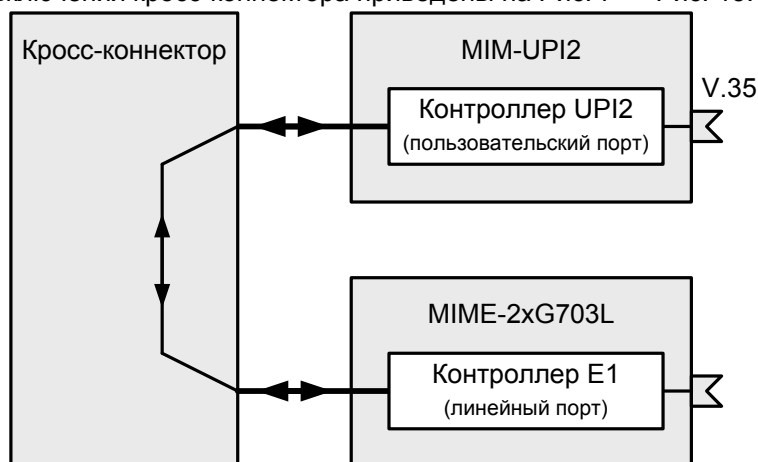
Рис. 7. Передача данных V.35 через канал E1
