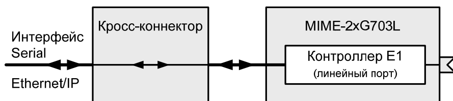
Рис. 9. Передача данных Ethernet/IP через выбранные таймслоты канала E1
