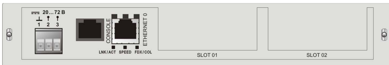
Рис. 24. Вид задней панели изделий MM-201x и MM-202x для установки в конструктивы P-12 и P-510 с питанием от сети постоянного тока
