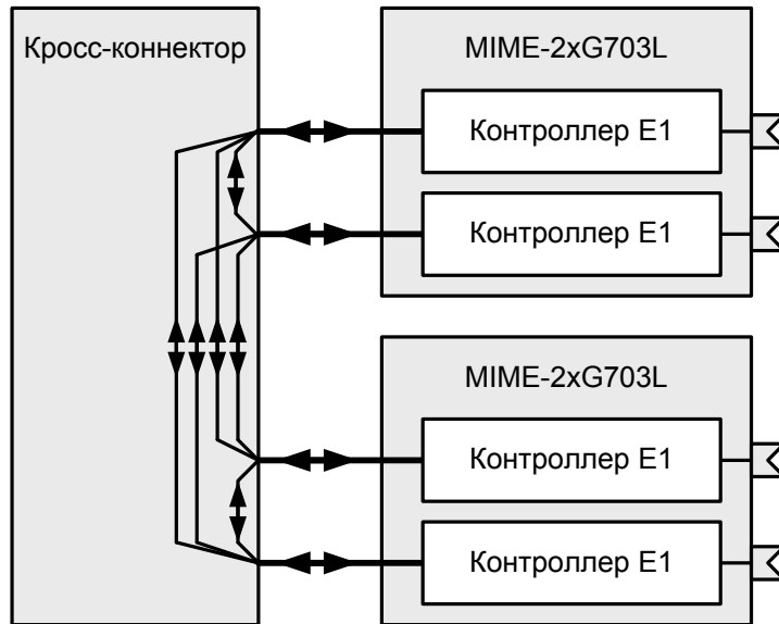
Рис. 11. Кросс-коммутация данных E1 между четырьмя потоками E1
