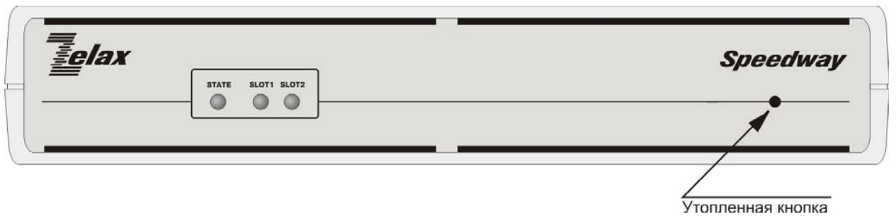
Рис. 16. Вид передней панели изделий MM-2xx настольного исполнения
