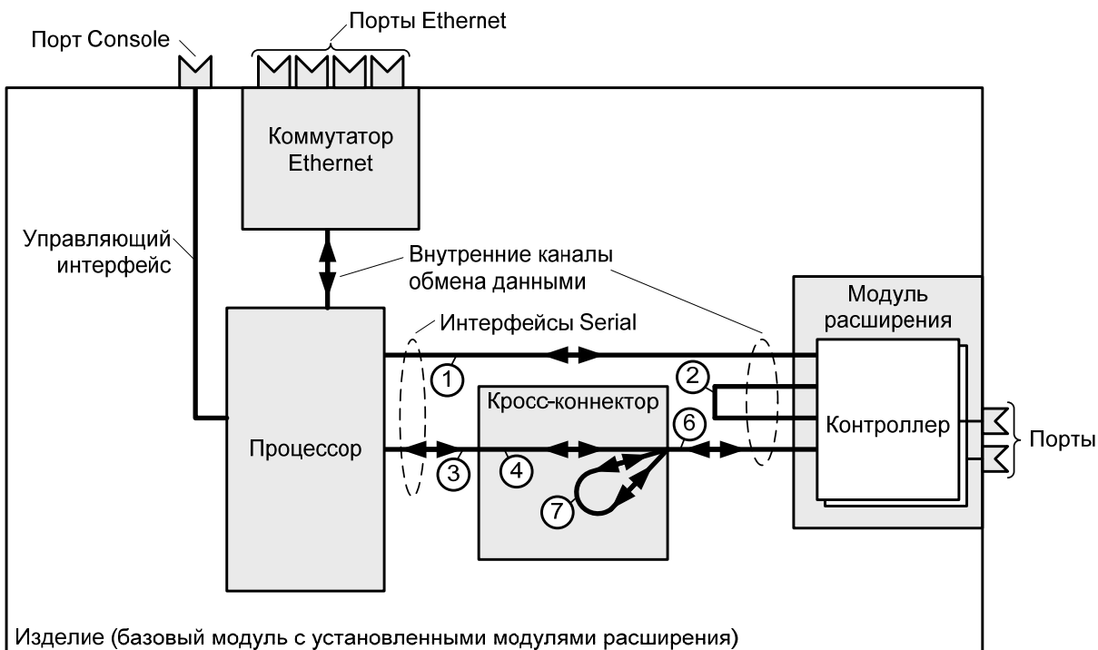
Рис. 6. Структурная схема изделия MM-205RC-UNI
